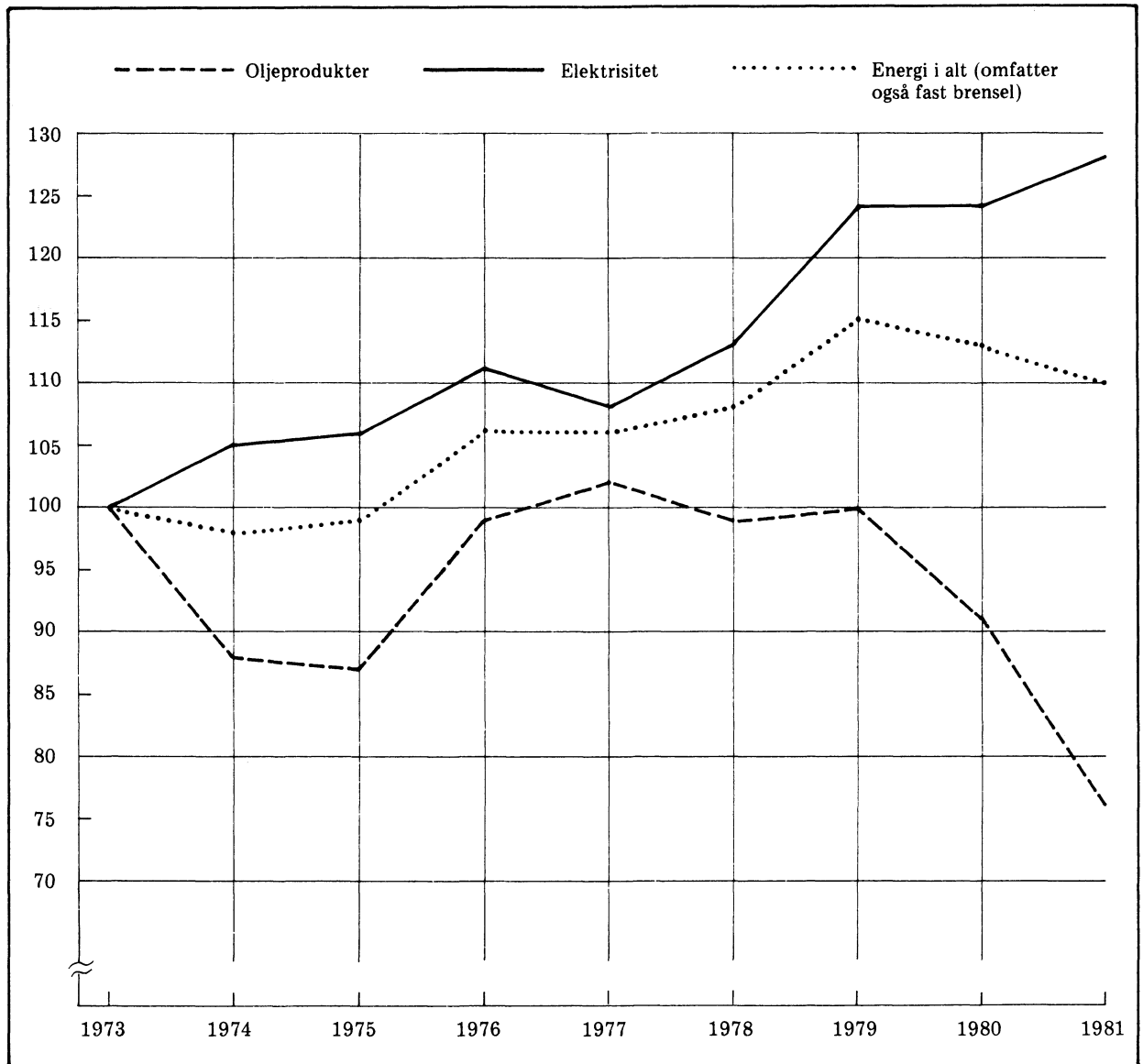
Figur 1. Bruk av oljeprodukter og elektrisitet til formål utenom råstoff og transport. Indeks 1973-1981 1973 = 100
