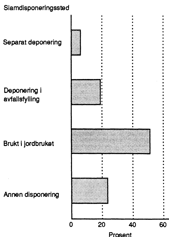
Figur 5. Avløpsrenseanlegg. Kjemikalieforbruk etter type. Prosent. 1991.
