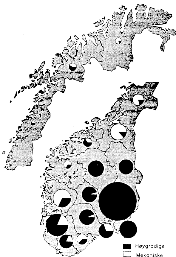
Figur 2. Avløpsrenseanlegg. Hydraulisk kapasitet (P.E.) fordelt på mekaniske og høygradige avløpsrenseanlegg. Fylke. 1991.
